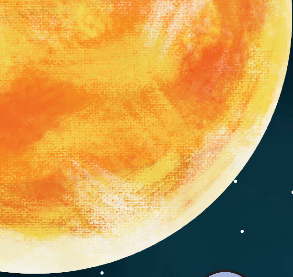
Słońce
