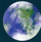
Ziemia
