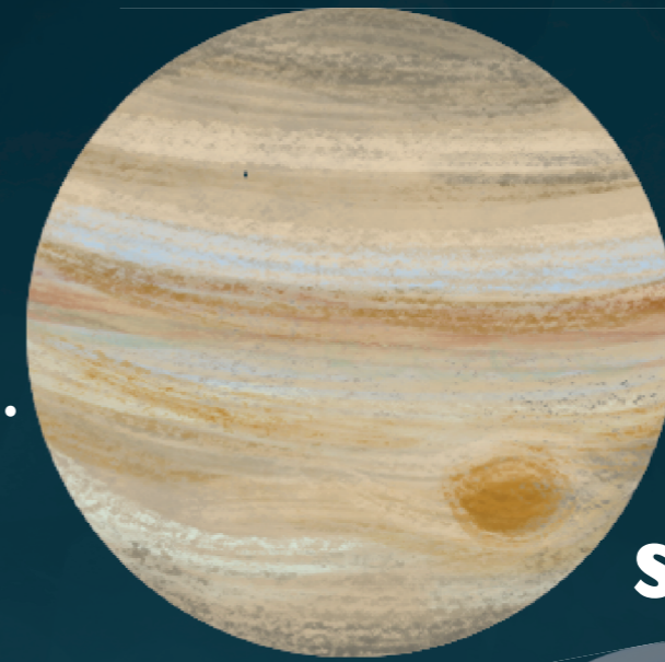
Jowisz
